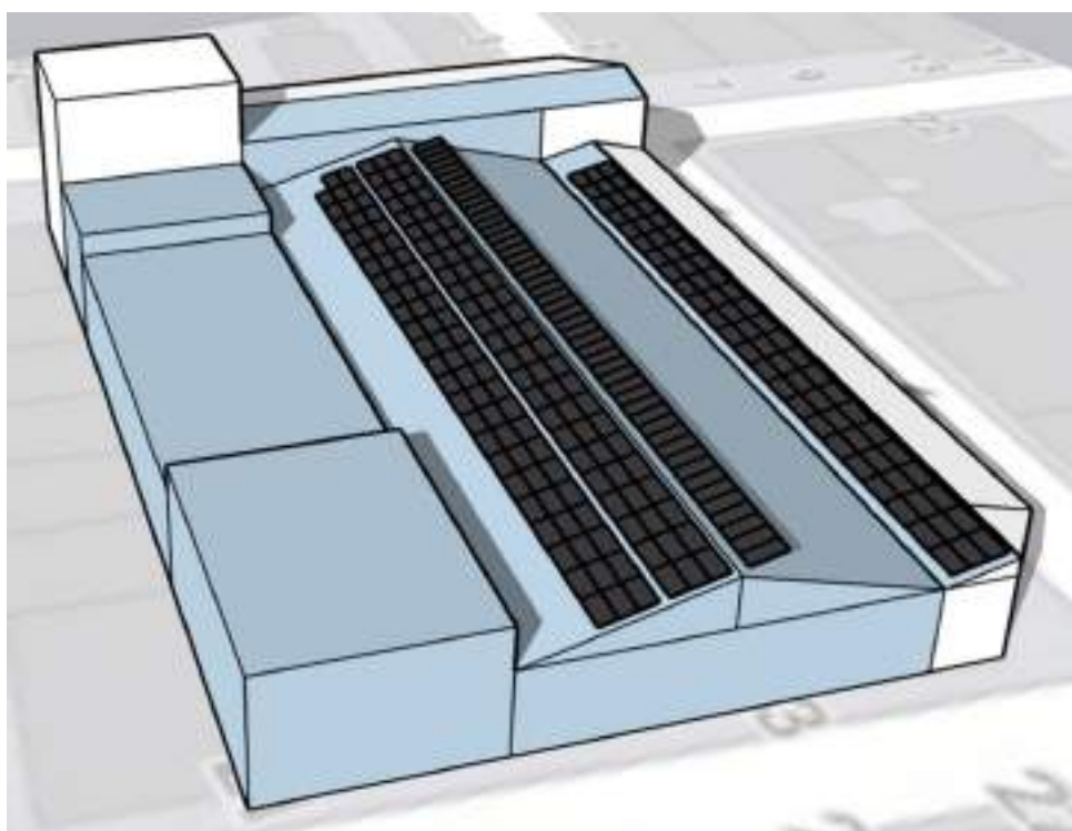
Figura 20: Implementación de la disposición de módulos fotovoltaicos en la cubierta de la nave de Fontcoop (Fuente: Grupo Enercoop).
