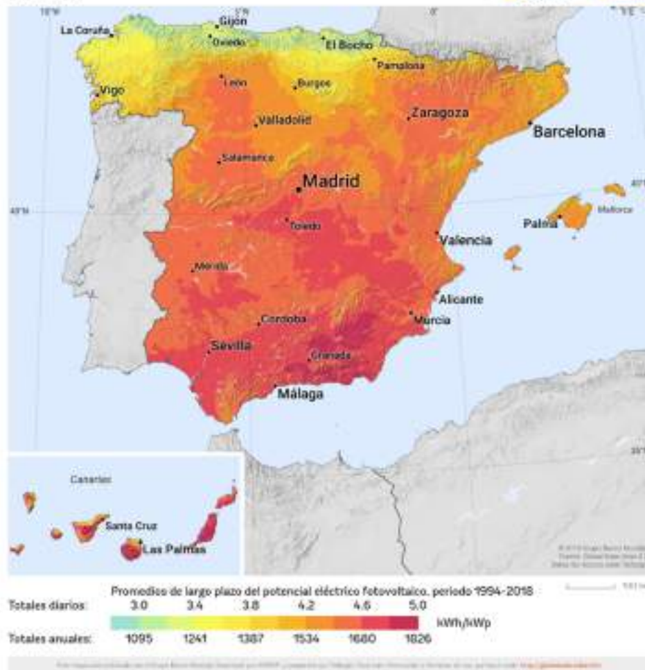
Figura 8: Mapa de radiación solar en España (Fuente: Global Solar Atlas / Solargis).
