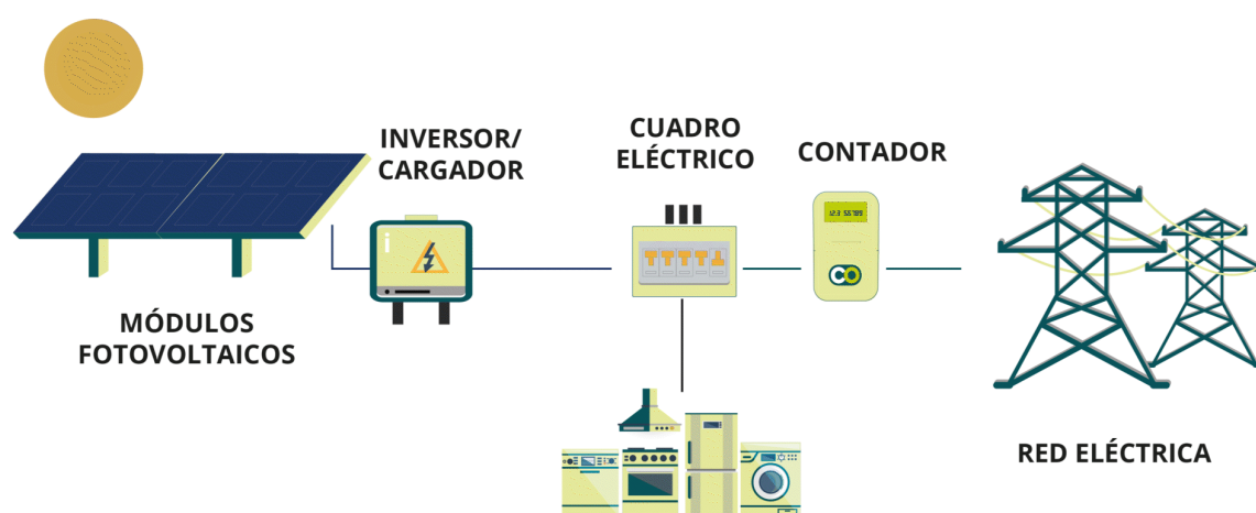
Figura 9: Esquema típico de una instalación de autoconsumo. (Fuente: Grupo Enercoop).
