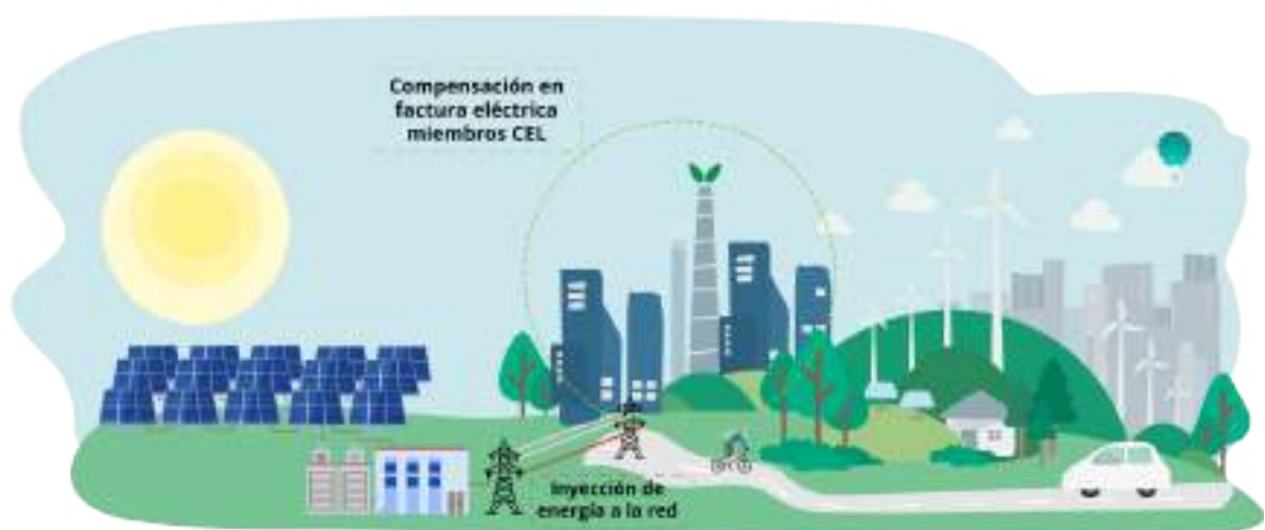
Figura 11: Esquema conceptual de plantas de producción asociadas a una comunidad energética (Fuente: Grupo Enercoop).
