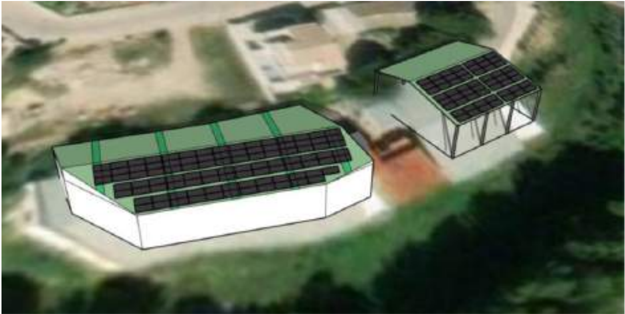
Figura 24: Simulación de la disposición de módulos fotovoltaicos en la cubierta de las naves de la cooperativa El Progreso (Bicorp - Valencia) (Fuente: Grupo Enercoop).
